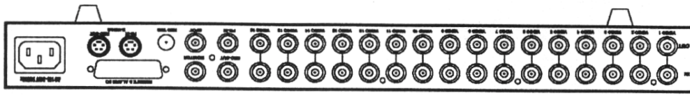
6-2 Vista esterna e dimensioni multiplexer MX162C
