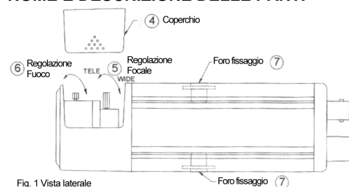
Fig. 1 Vista laterale
