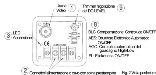
Fig. 2 Vista posteriore
