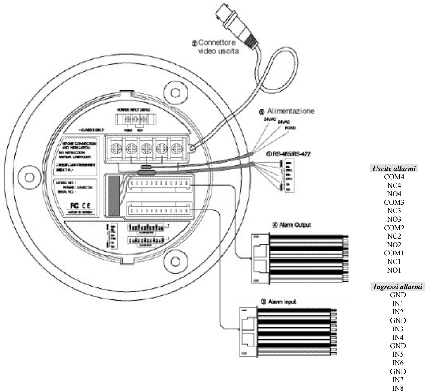
[Fig.10a] – Schema delle connessioni GCP-7425D.
