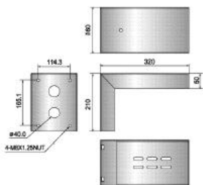
DIMENSIONI
