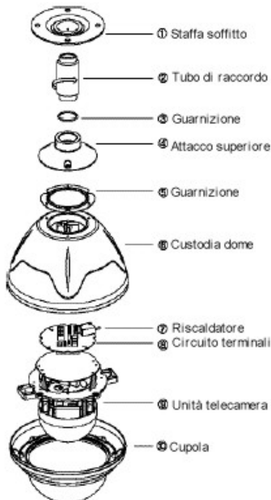
[Fig.1a] – Lista delle parti
