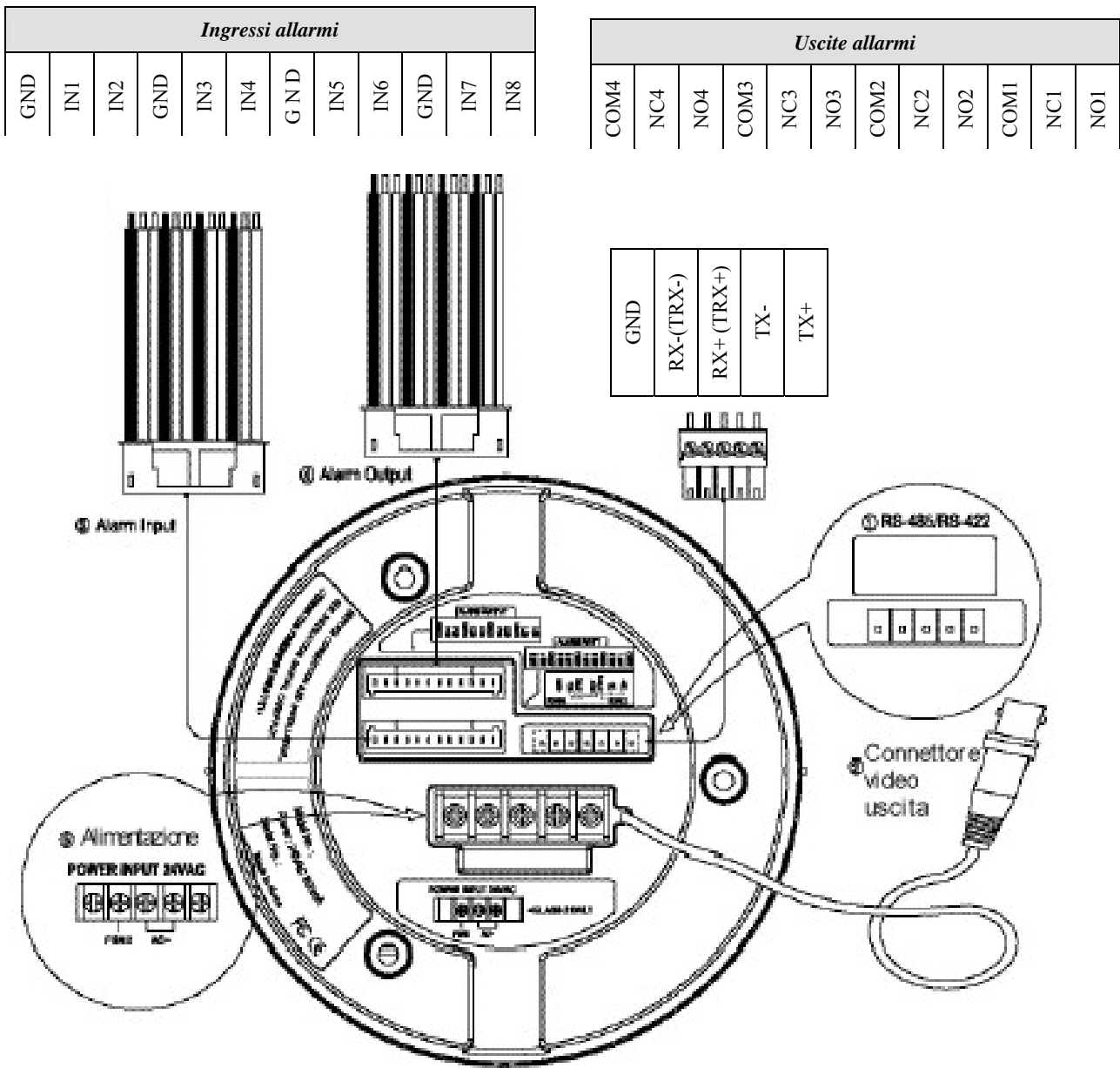
[Fig.10b] – Schema delle connessioni GHSD-7425D.
