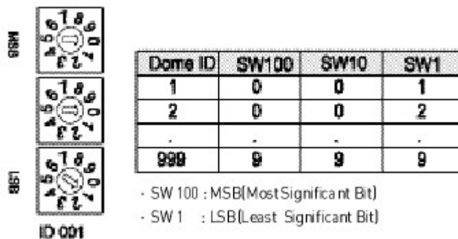
[Fig.9] – Settaggio indirizzo (ID) della telecamera.
