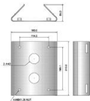
DIMENSIONI
