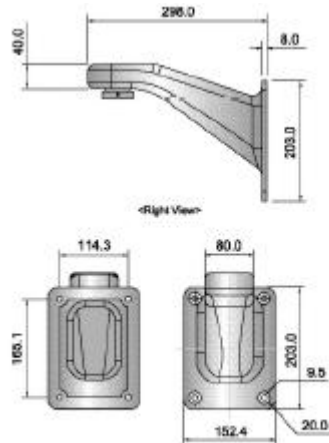
DIMENSIONI
