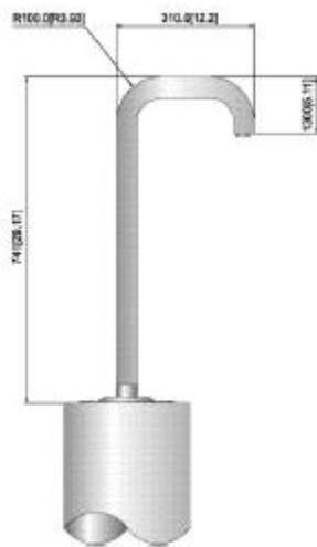
DIMENSIONI
