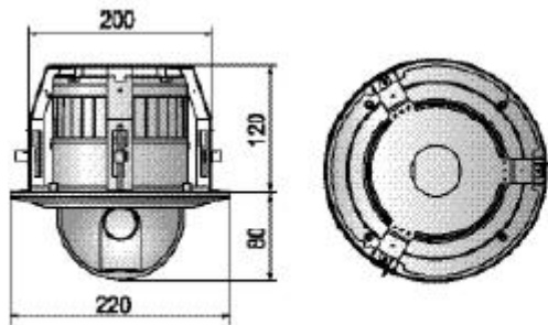
DIMENSIONI
