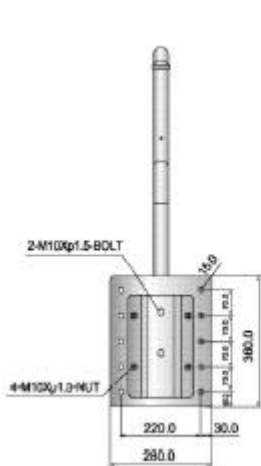
DIMENSIONI
