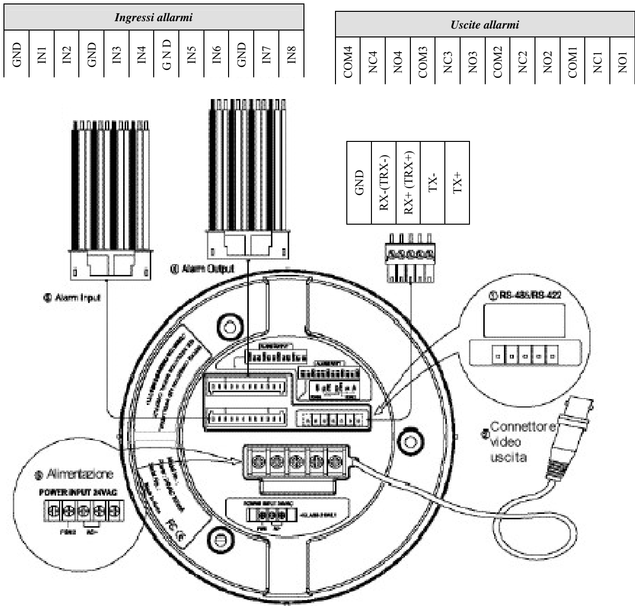
[Fig.10b] – Schema delle connessioni GHSD-7436D.
